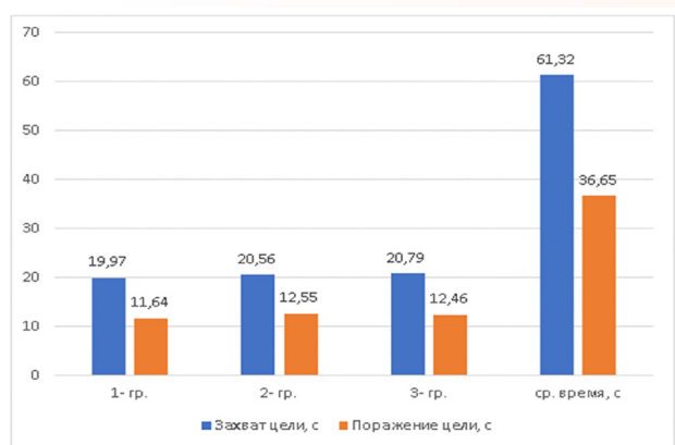
Рис.5. Среднее время захвата и поражения цели 1, 2 и 3 групп характеризующая мобильность (подвижность) стрелков при выполнении упражнения.
