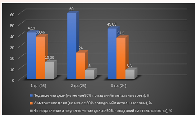
Рис.3. Степень поражения цели 1, 2 и 3 групп (%)
