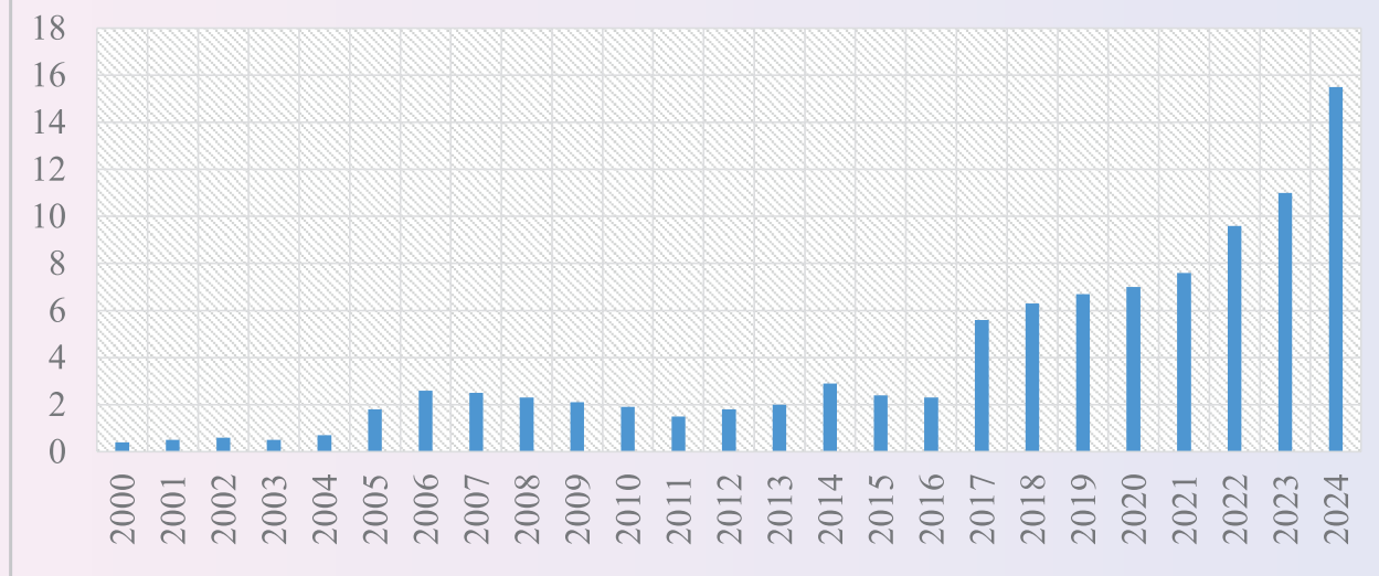
1- rasm. Yillar kesimida aniqlangan yangi zaifliklarning ulushi (CVE)
