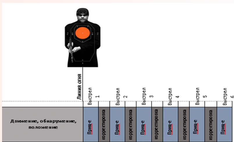
Рис. 4. Визуальное представление измерений захвата цели (т. е. движение, обнаружение, положение) и поражения цели (т. е. прицеливание, стрельба, корректировка, прицеливание, стрельба и т. д.) для поражения каждой цели.
