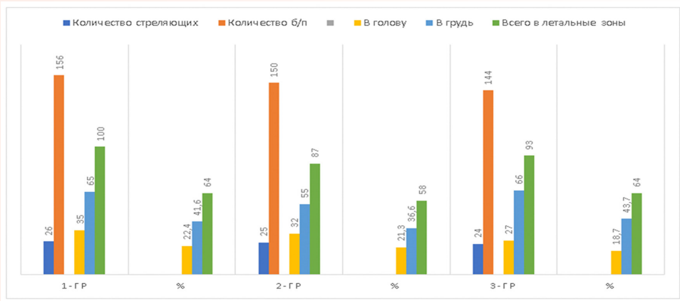
Рис. 1. Данные результатов стрельбы в летальные зоны цели
