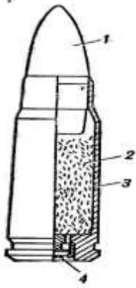
117-расм. Жанговар патроннинг кўриниши
