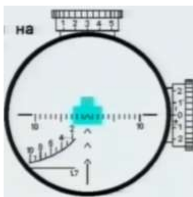
182-расм. Мўлжалга олиш мосламасидан тўғри мўлжалга олиш ҳолати.
