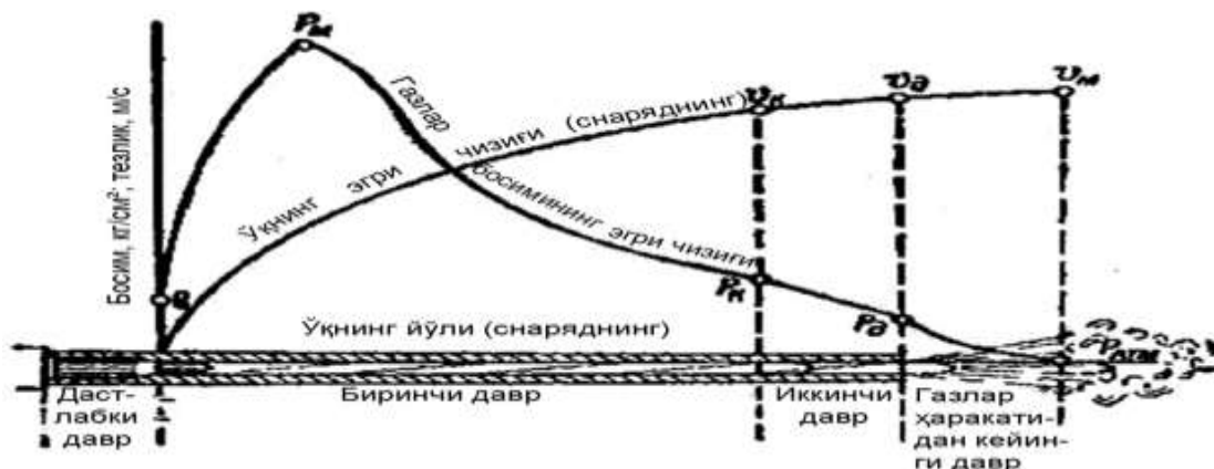
1-расм. Ўқ отилганида содир бўладиган 4 та босқич.
