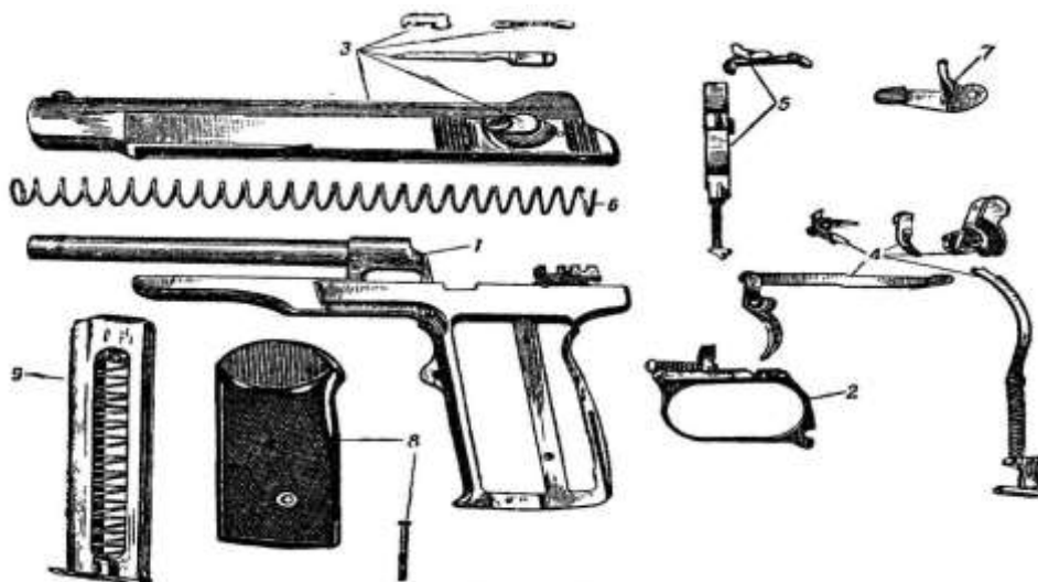
49-расм: Пистолетнинг асосий қисм ва механизмлари:
