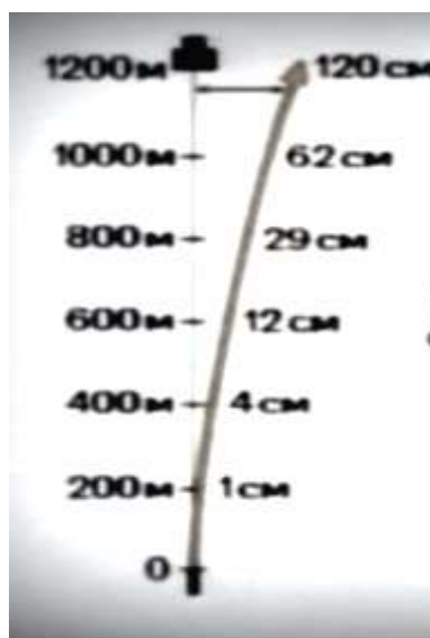
183-расм. СВД дан отилган ўқ деривация (стволдаги қирқимлар сабабли ўқнинг ўнг томонга айланиши) ҳисобига нишондан масофага қараб ўнг томонга огиши.
